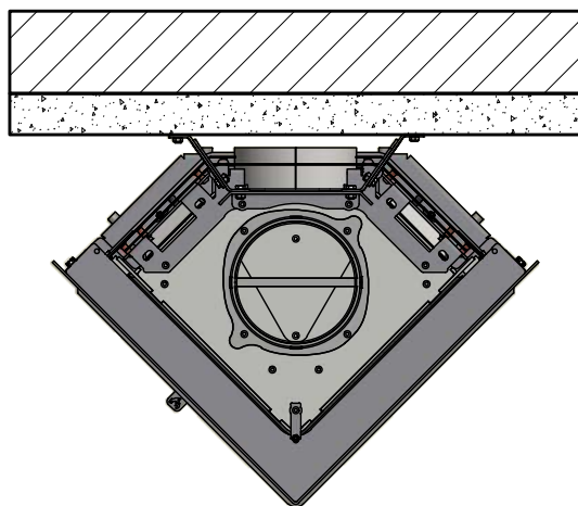
Fastsättning parallellt
