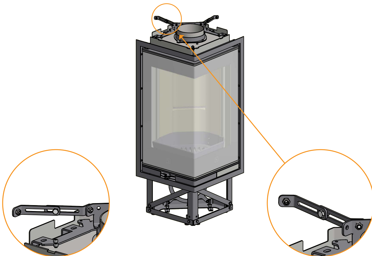
Fastsättning hörn
