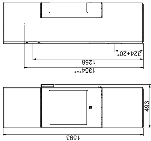
Scanspis 84 (Modern Maxi och Classic Maxi)
