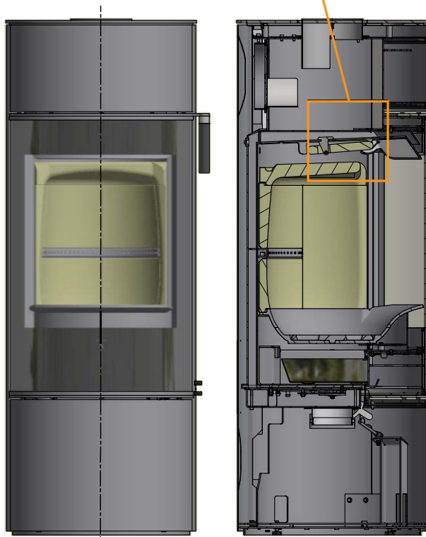
Hållare för den översta rökvändarplattan
