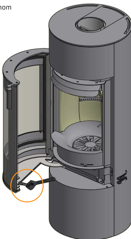
Låsmekanisme
