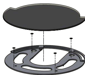
Glasplatta för bakutgång
